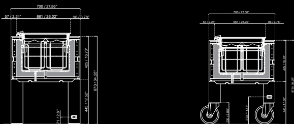
Tavolo BELLEVUE con vasca PANORAMA senza riserva BELLEVUE table with PANORAMA tank with one level of gelato tubs Table BELLEVUE avec cuve PANORAMA sans réserve BELLEVUE Theke mit PANORAMA-Wanne ohne Vorrat Mesa BELLEVUE con cuba PANORAMA sin reserva
