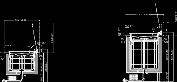
Vasca da incasso PANORAMA senza riserva PANORAMA built-in tank with one level of gelato tubs Cuve PANORAMA encastrable sans réserve Einbaus-PANORAMA-Wanne für Gelato/Granita ohne Vorrat Cuba PANORAMA empotrada sin reserva
