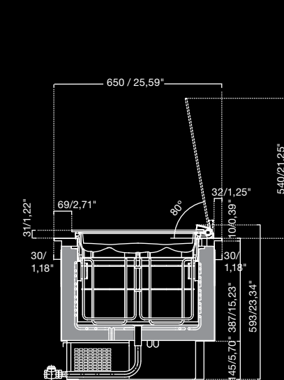
Vasca da incasso PANORAMA senza riserva PANORAMA built-in tank with one level of gelato tubs Cuve PANORAMA encastrable sans réserve Einbau-PANORAMA-Wanne für Gelato/Granita ohne Vorrat Cuba PANORAMA empotrada sin reserva
