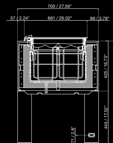
Tavolo BELLEVUE con vasca PANORAMA senza riserva BELLEVUE table with PANORAMA tank with one level of gelato tubs Table BELLEVUE avec cuve PANORAMA sans réserve BELLEVUE Theke mit PANORAMA-Wanne ohne Vorrat Mesa BELLEVUE con cuba PANORAMA sin reserva
